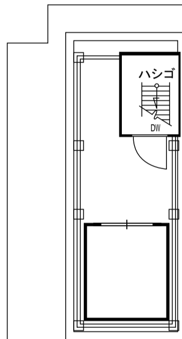
〈屋上平面図〉
